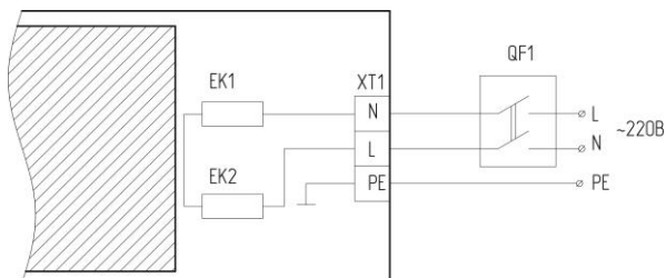
Рисунок 2. Обогреватель ИН-2.0
